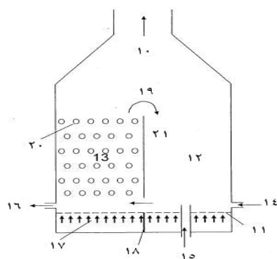
شكل ٣ منظر تخطيطي لنموذج مثالي لجهاز التحبيب وفقاً للاختراع
